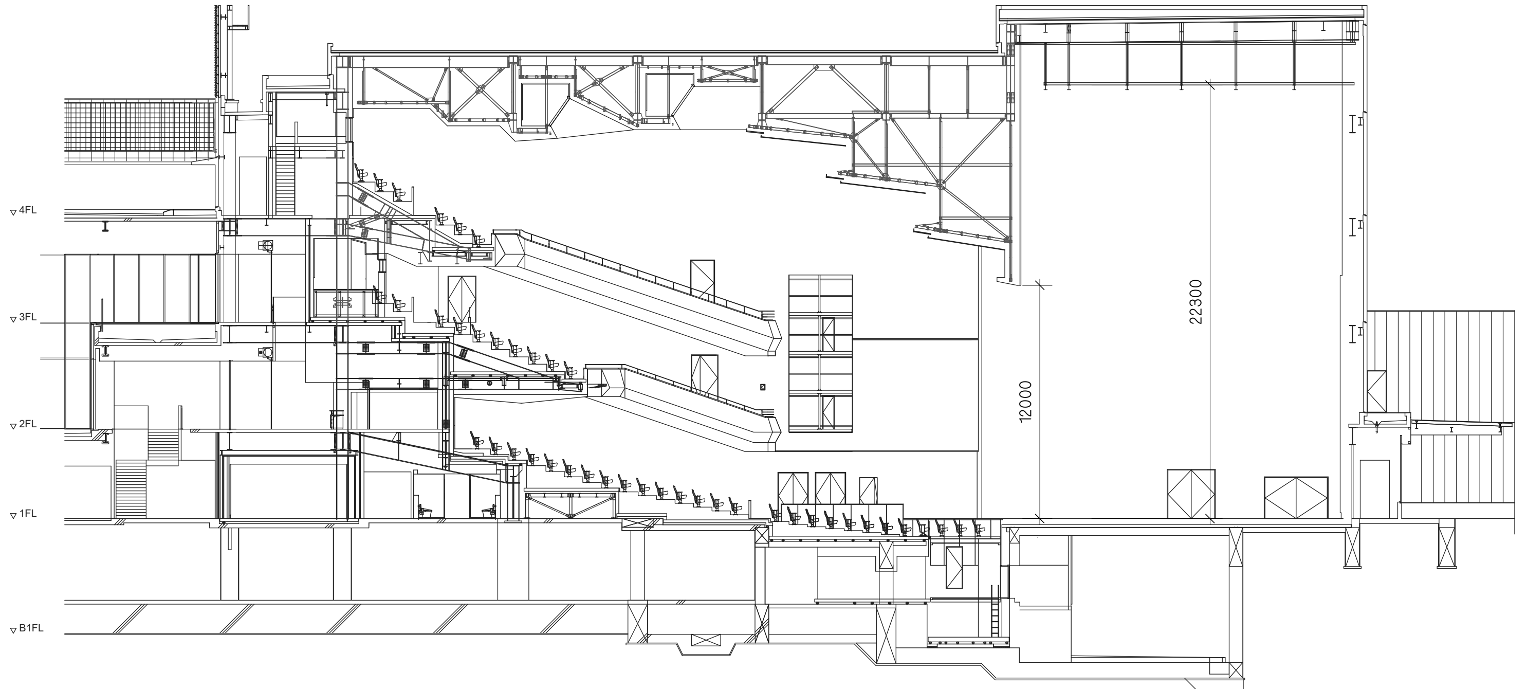
ホール断面図 S=200:1
