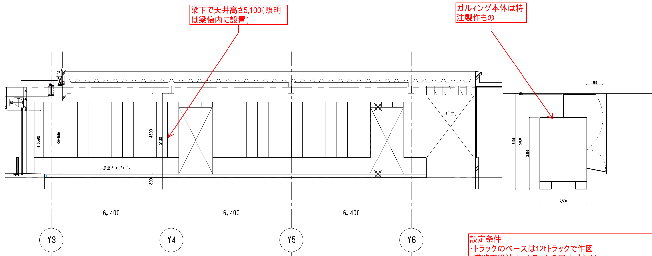
ホール棟荷捌き室断面図 1/100
