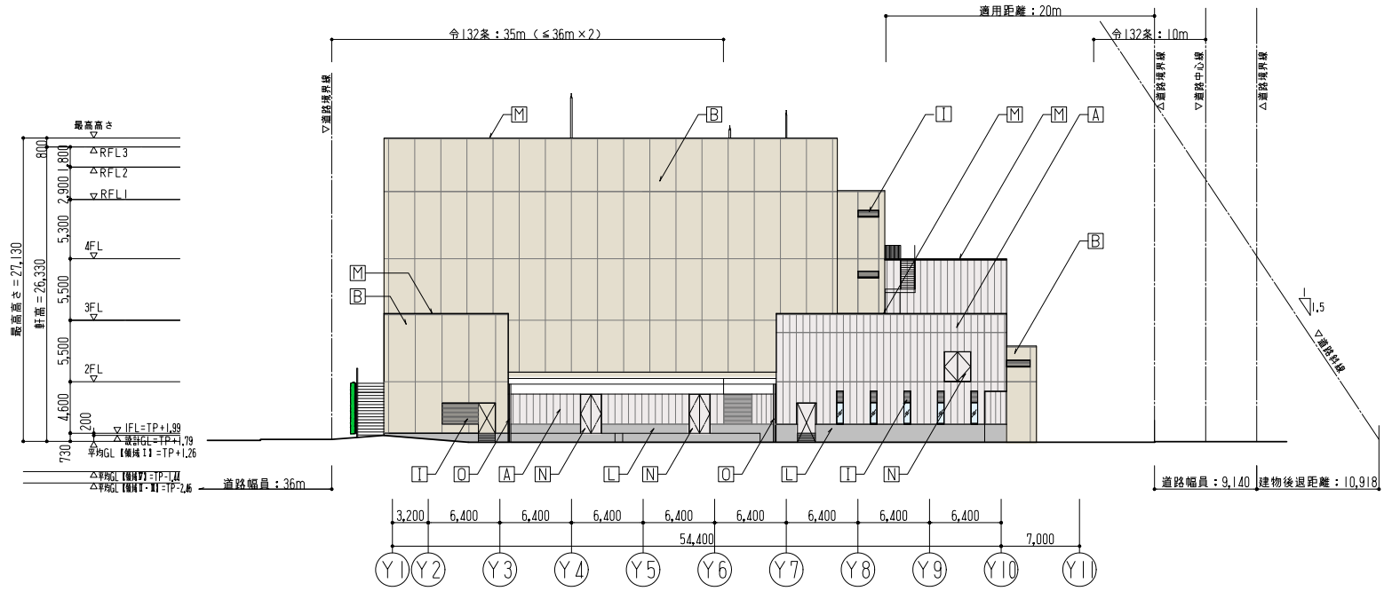
東側立面図
