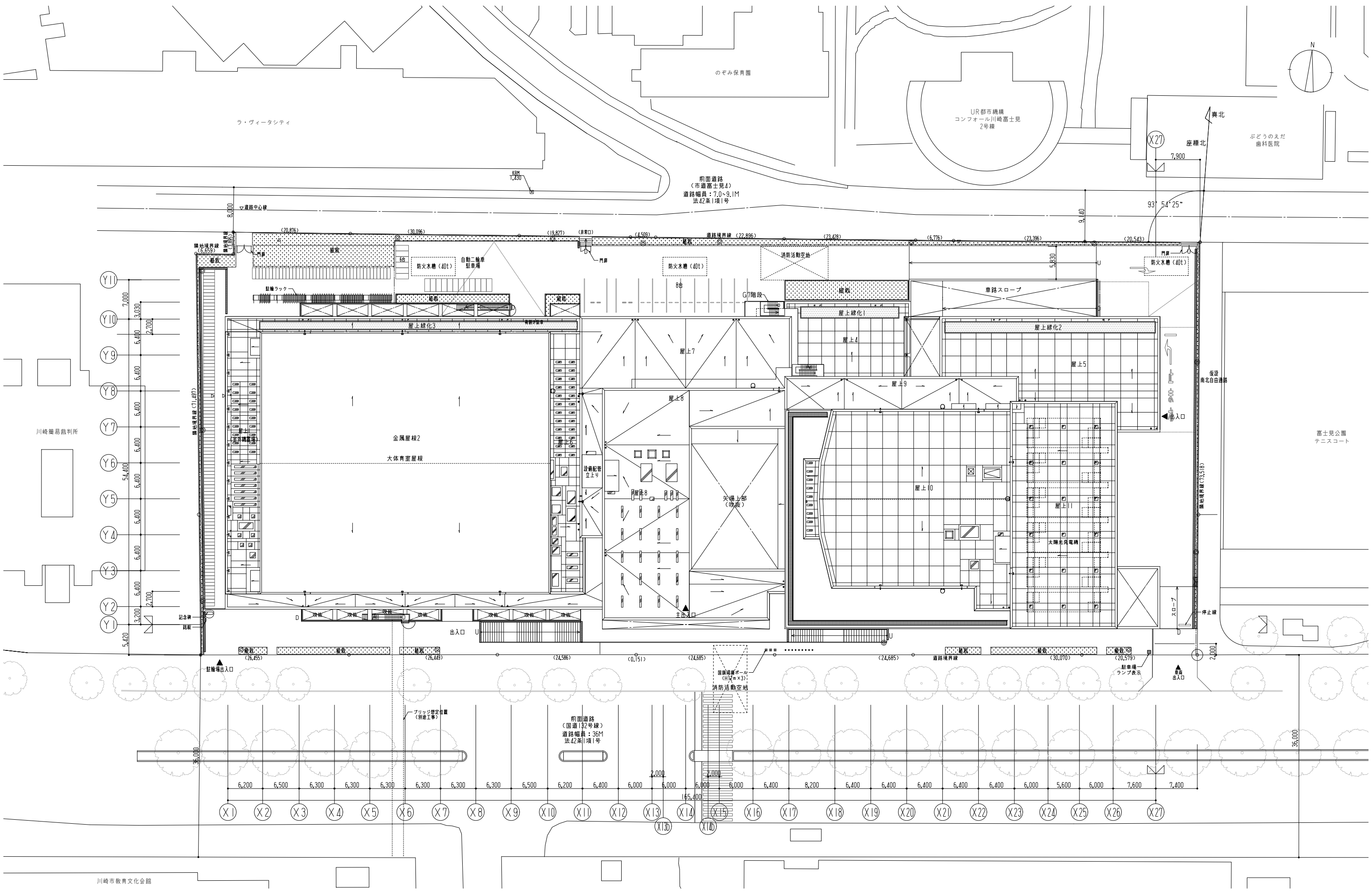
配置図 兼 屋根伏図
